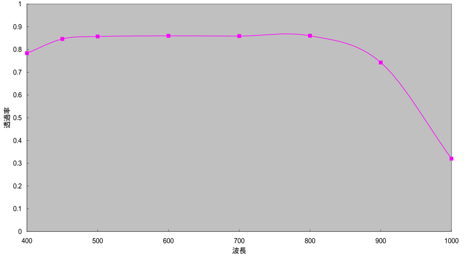
LM8JC10M 透過率
