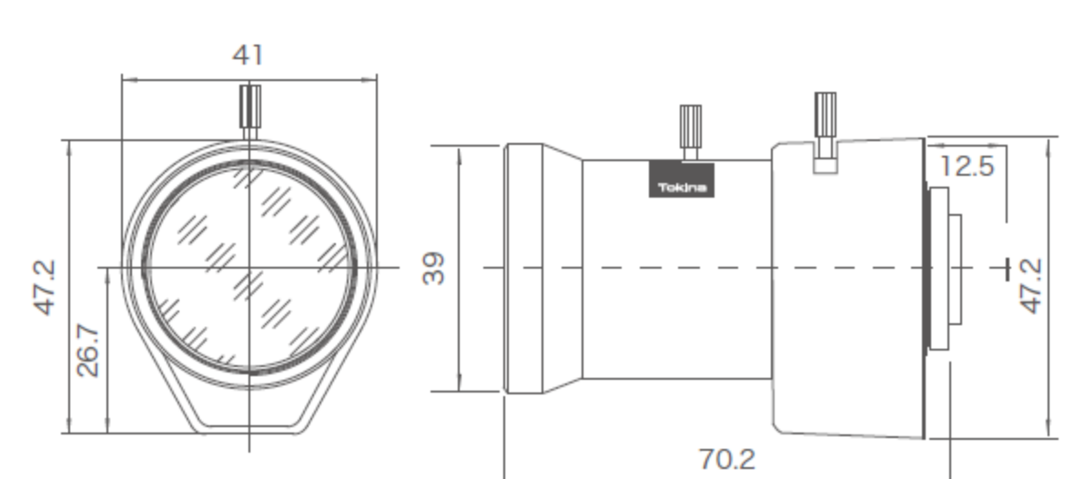
TVR0516HDDC-IR
