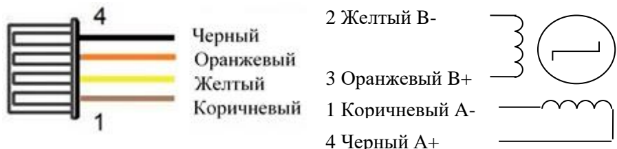
Схема подключения
